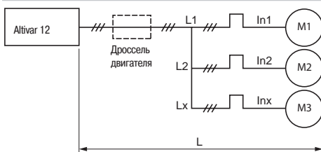
Параллельное подключение двигателей
