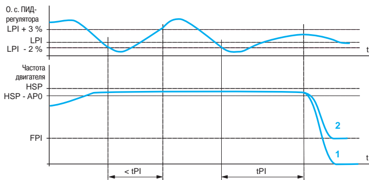
Контроль обратной связи ПИД-регулятора
