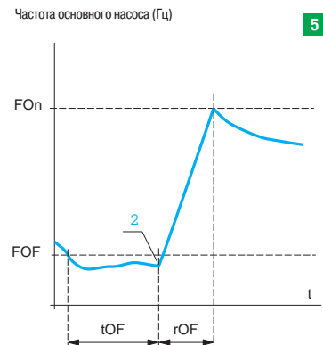
Остановка вспомогательного насоса
